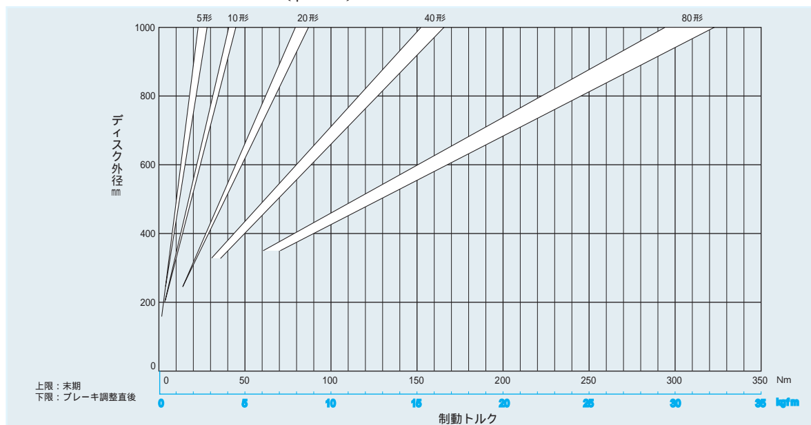
NGB形 ディスク外径・制動トルク曲線( \mu=0.33 )
