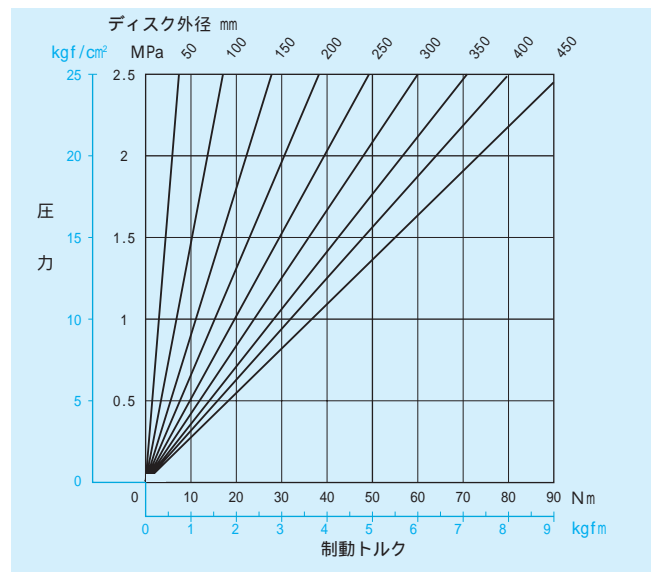
DBL-50、RDB-50 圧力・制動トルク曲線（ \mu=0.33 ）
