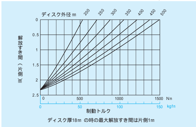
NDB-1400A形 解放すき間 (片側)・制動トルク曲線(μ=0.33)
