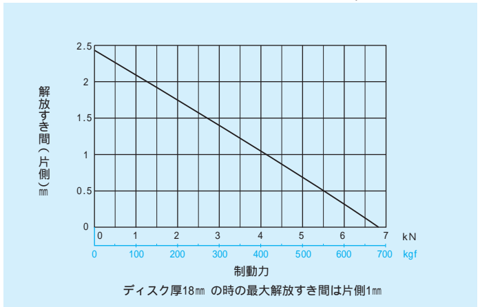
NDB-1400A形 解放すき間 (片側)・制動力曲線(μ=0.33)
