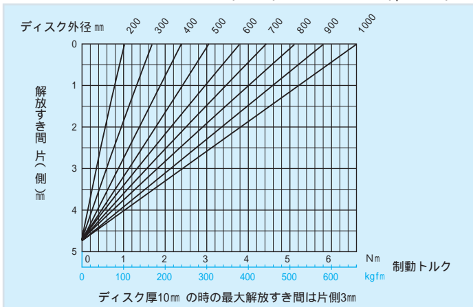
NDB-1400B形 解放すき間 (片側)・制動トルク曲線(μ=0.33)
