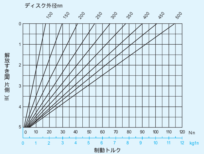
NDB-20A形 初期解放すき間(片側)・制動トルク曲線(μ=0.35)
