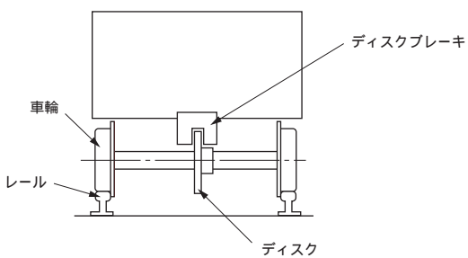
走行車両の制動およびパーキング。 構内走行車、遊園地施設、トロッキなど。
