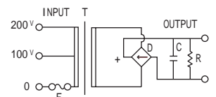
回路図
