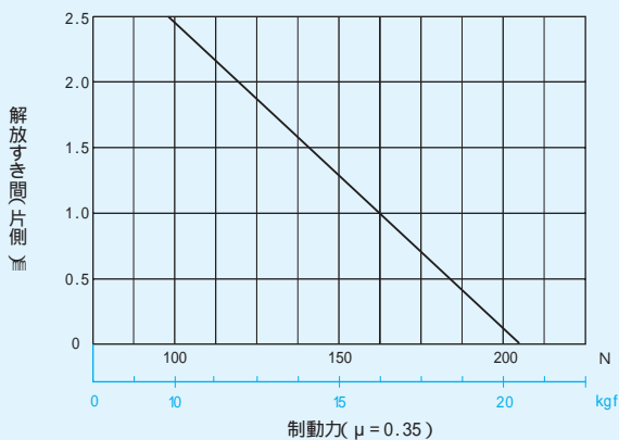
NDB-10A形 初期解放すき間(片側)・制動力曲線(μ=0.35)
