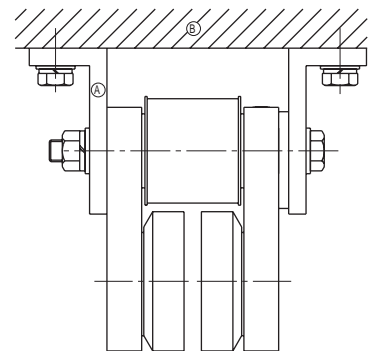
A、B共に磁性体の場合、非磁性体のワッシャーを片側にはさみ込む
