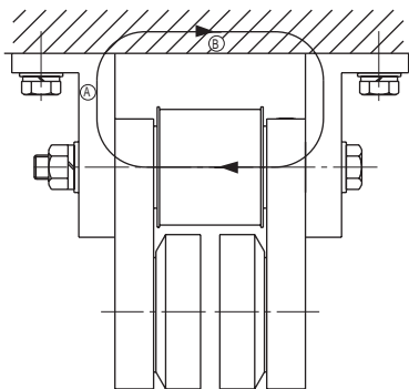
A、B共に磁性体の場合には磁束が短絡し、制動力が出ない
