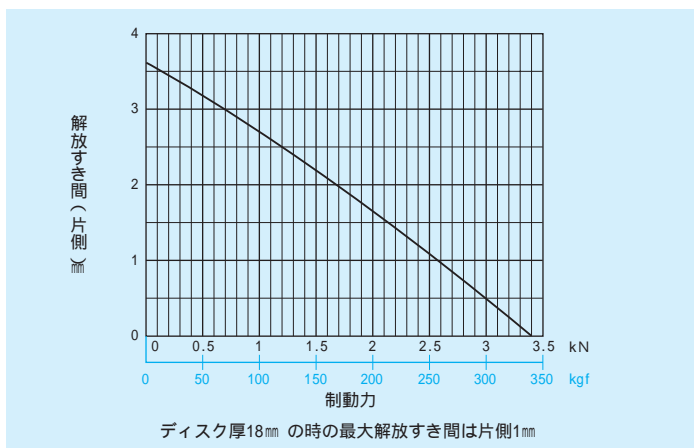
NDB-400B形 解放すき間 (片側)・制動力曲線(μ=0.33)
