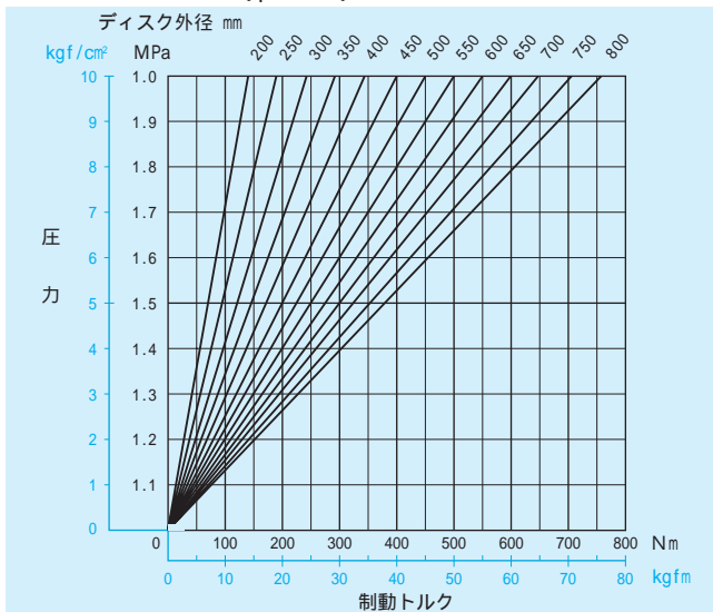
DBA-100、DBL-100 圧力・制動トルク曲線（ \mu=0.33 ）
