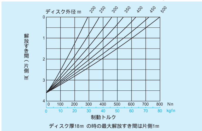
NDB-400B形 解放すき間 (片側)・制動トルク曲線(μ=0.33)
