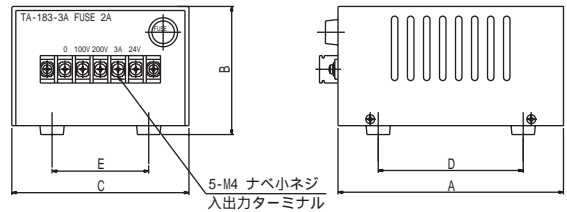
外形図
