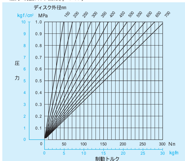
DBA-20、DBL-20、RDB-20 圧力・制動トルク曲線(μ=0.33)
