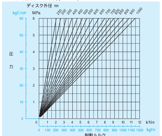
DBL-100 圧力・制動トルク曲線（ \mu=0.33 ）
