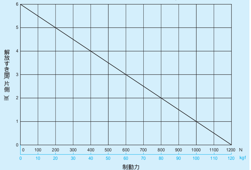
NDBA-50形 解放すき間 (片側)・制動力曲線(μ=0.35)
