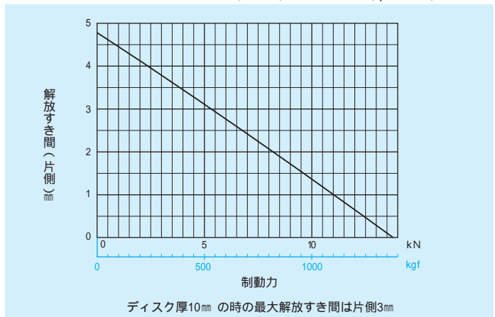
NDB-1400B形 解放すき間 (片側)・制動力曲線(μ=0.33)
