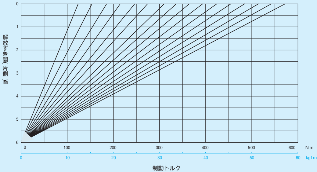
NDBA-50形 解放すき間 (片側)・制動力曲線(μ=0.35)
