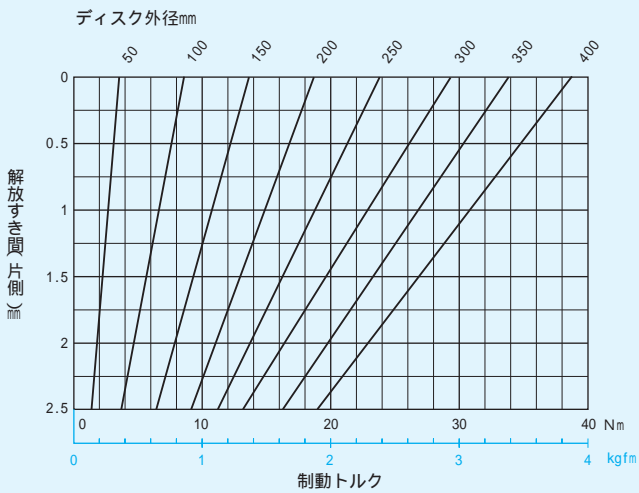
NDB-10A形 初期解放すき間(片側)・制動トルク曲線(μ=0.35)
