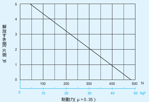
NDB-20A形 初期解放すき間(片側)・制動力曲線(μ=0.35)
