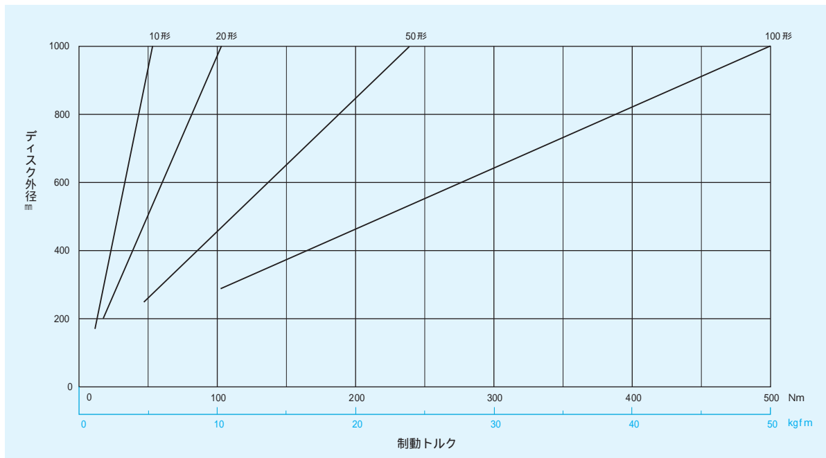
NGDB形 ディスク外径・制動トルク曲線( \mu=0.33 )
